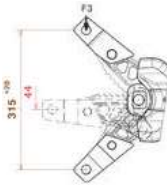
Zugaufsatz Teile-Nr. 2836033
